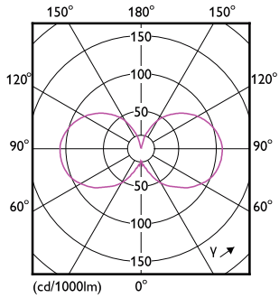
LEDLuster MAS SLR P45 2,5W E14 927 CL-LDD
