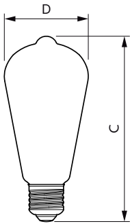
Bulb ST64 EU 6-60W 810lm WG E27 CL
