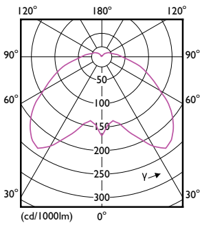
LEDcandle MAS SLR1 B40 8W E14 827 CL-LDD
